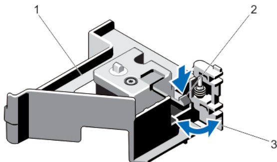
图 21: 打开和关闭 PCIe 卡固定器门锁
