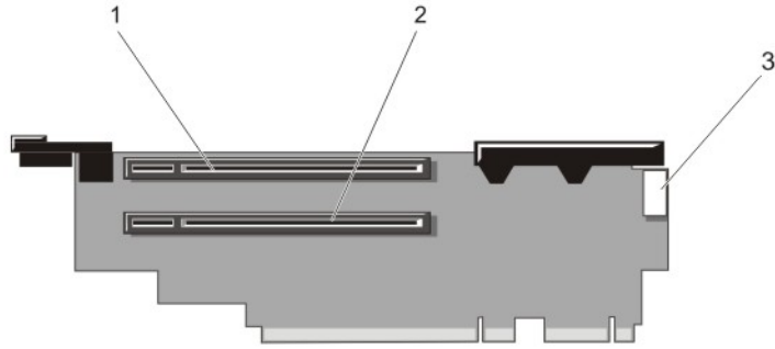
图 30: 识别扩充卡提升板 3 上的连接器
