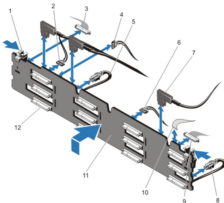
图 42: 卸下和安装 3.5 英寸 (x12) SAS/SATA 背板
