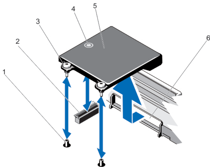
图 35: 卸下和安装网络子卡
