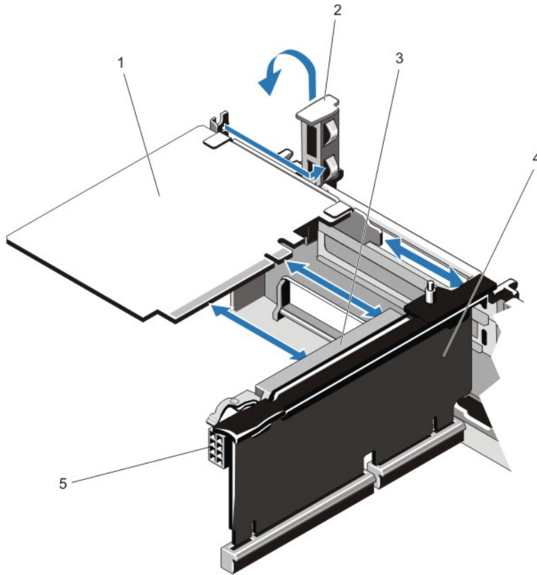
图 23: 卸下和安装扩充卡
