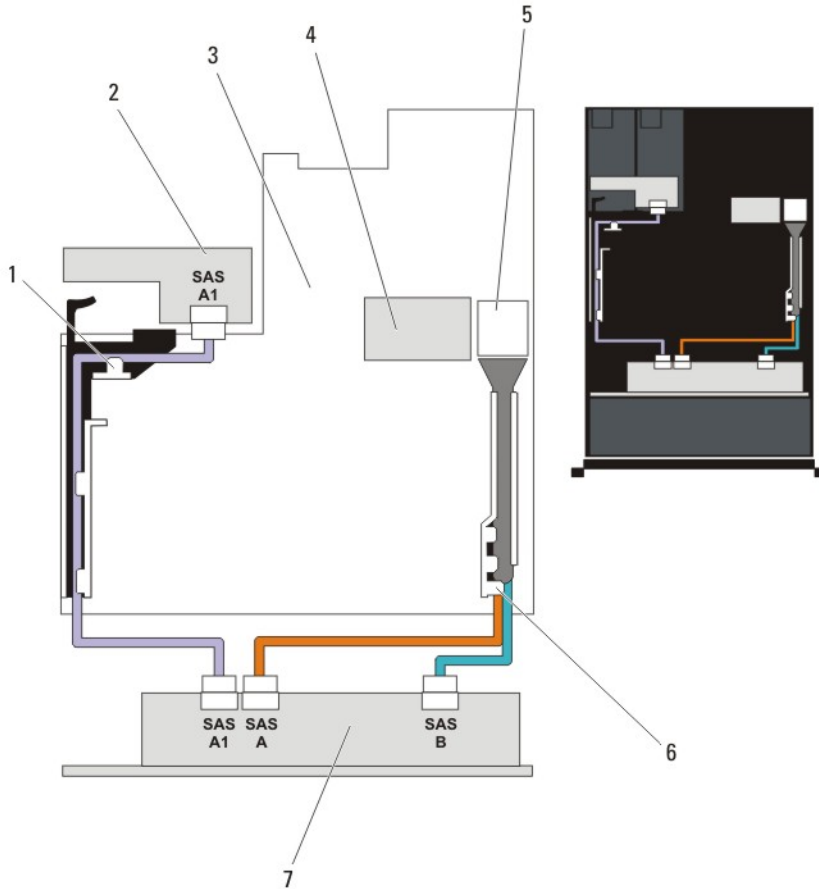
图 45: 布线图—2.5 英寸 (x2) 硬盘驱动器背板（背面）
