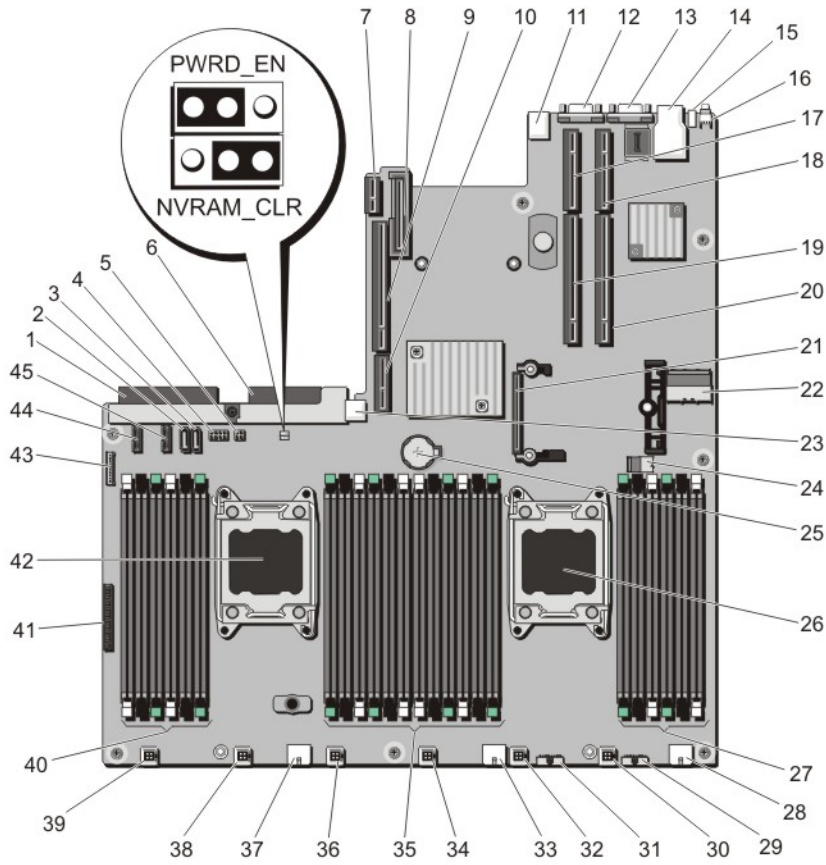
图 49: 系统板跳线和连接器
