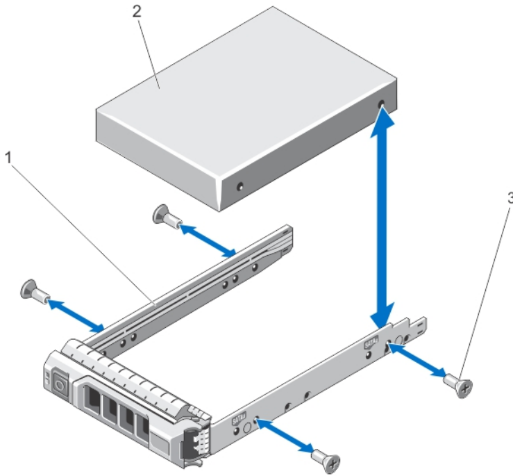
图 16: 在硬盘驱动器托盘中卸下和安装硬盘驱动器
