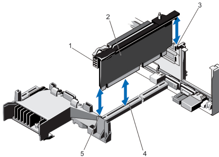
图 27: 卸下和安装扩充卡提升板 2
