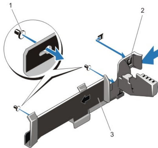
图 22: 卸下和安装电缆固定支架
