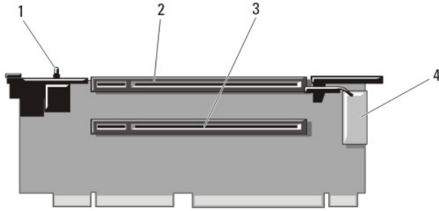
图 28: 识别扩充卡提升板 2 上的连接器
