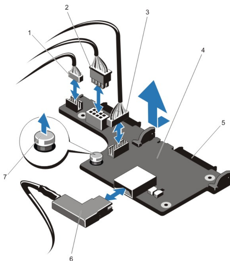
图 44: 卸下和安装 2.5 英寸 (x2) 硬盘驱动器背板（背面）
