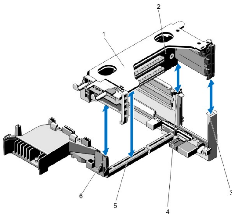
图 25: 卸下和安装扩充卡提升板 1
