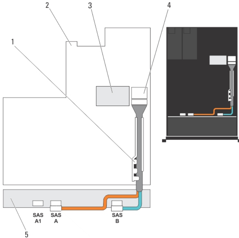
图 43: 布线图—3.5 英寸 (x12) SAS/SATA 背板
