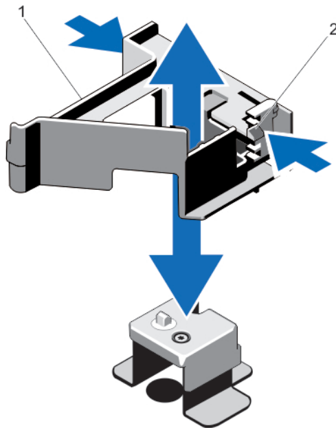
图 20: 卸下和安装 PCIe 卡固定器
