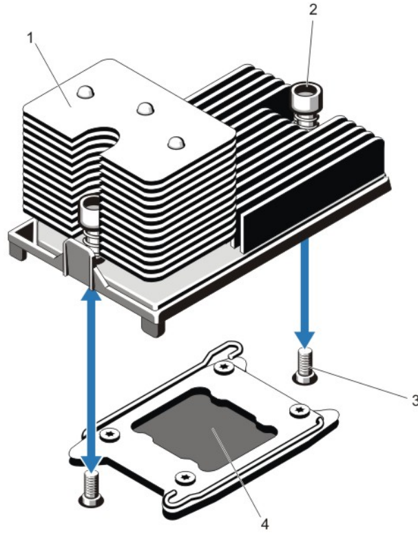
图 36: 卸下和安装处理器散热器
