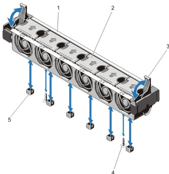
图 18: 卸下和安装冷却风扇部件
