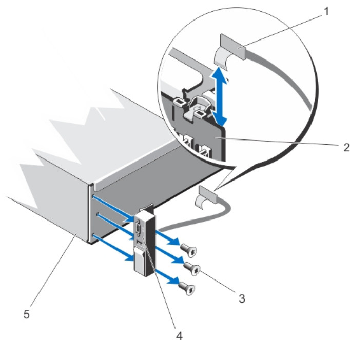
图 47: 卸下和安装 I/O 面板
