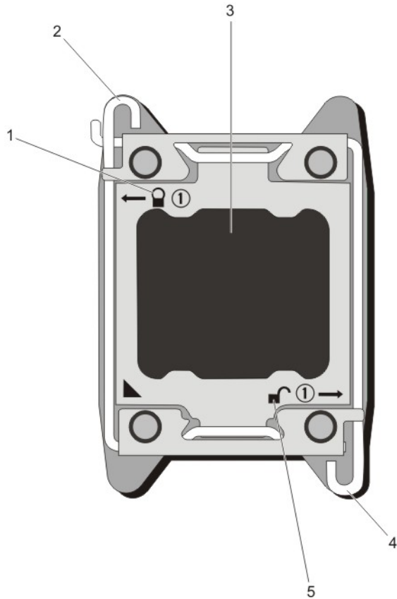
图 37: 处理器护盖打开与合上拉杆的顺序
