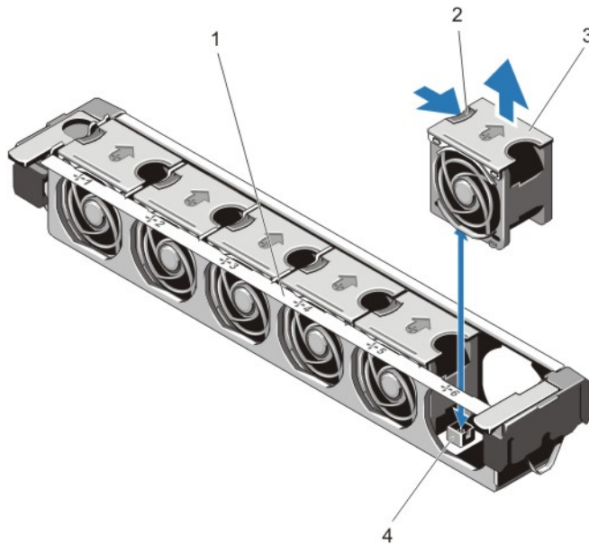
图 17: 卸下和安装冷却风扇
