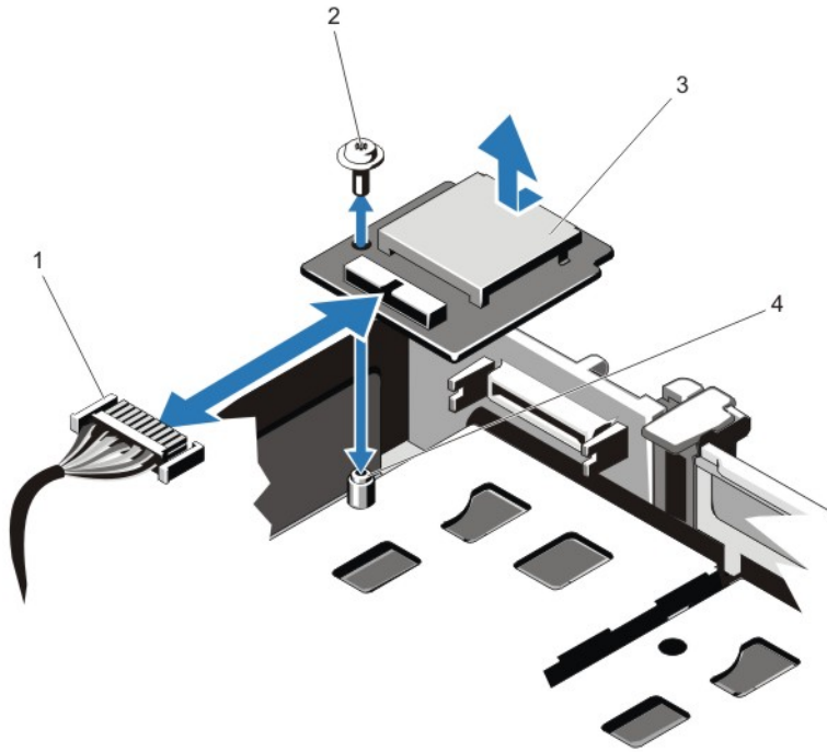
图 32: 卸下和安装 vFlash 介质单元
